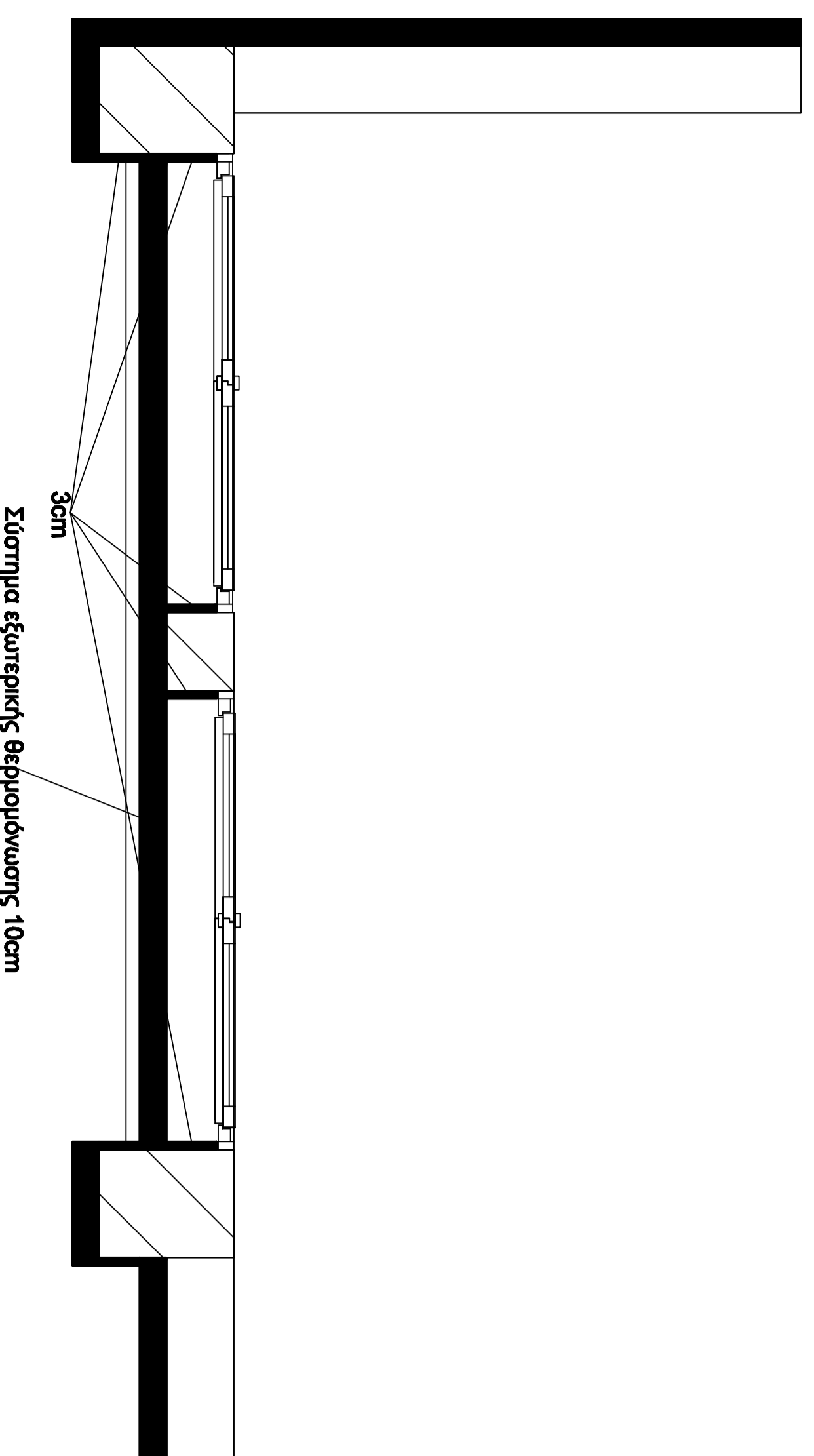
ΑΕΠΤΟΜΕΡΕΙΑ ΤΟΠΟΘΕΤΗΣΗΣ ΕΞΩΤΕΡΙΚΗΣ ΘΕΡΜΟΜΟΝΩΣΗΣ ΚΑ. 1:20
